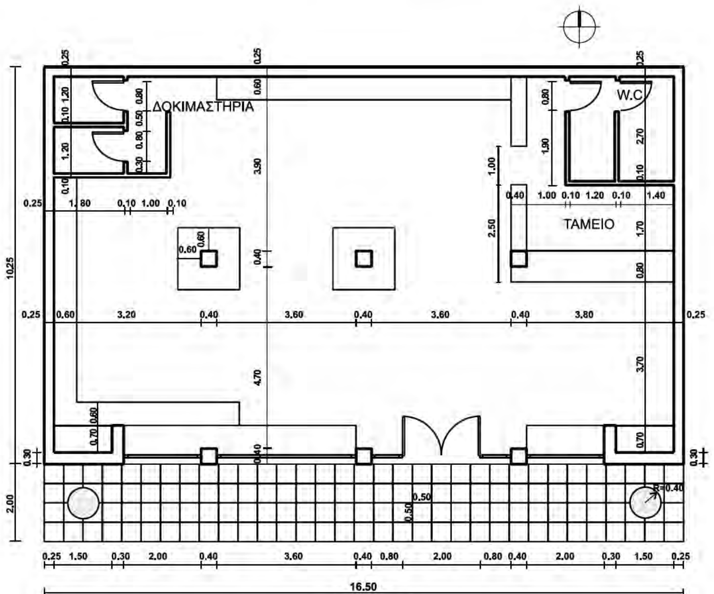
ΚΑΤΟΨΗ
