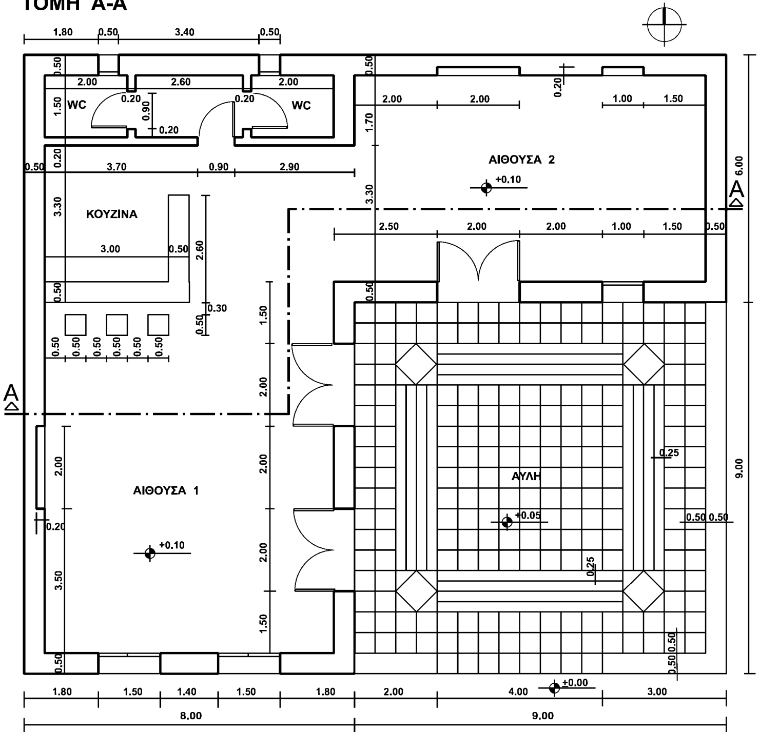
TOMH A-A
