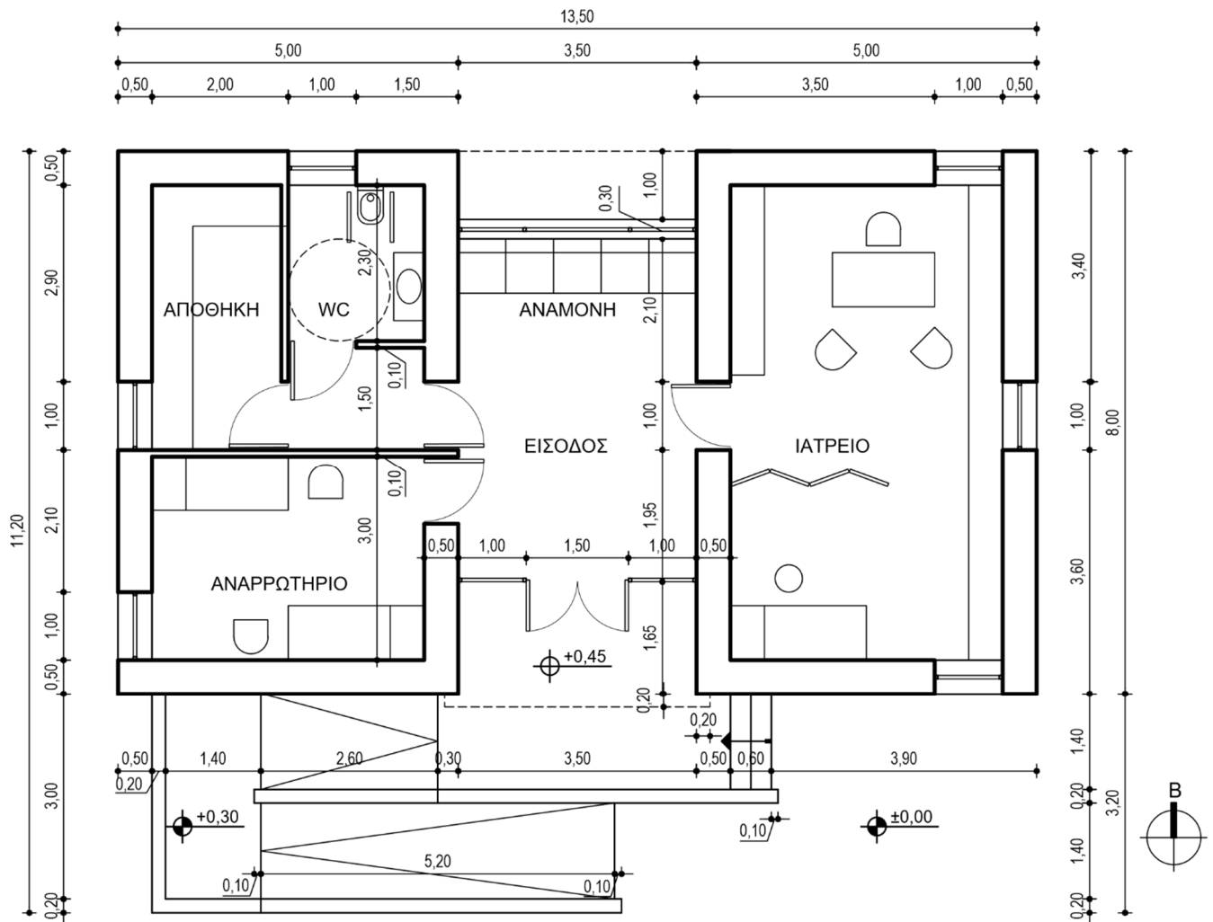
ΚΑΤΟΨΗ
