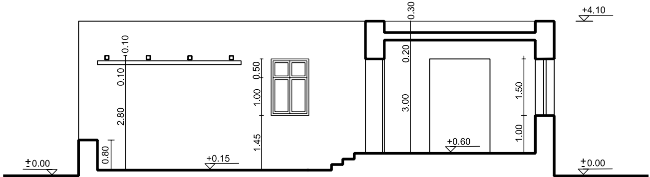
ΤΟΜΗ Α-Α
