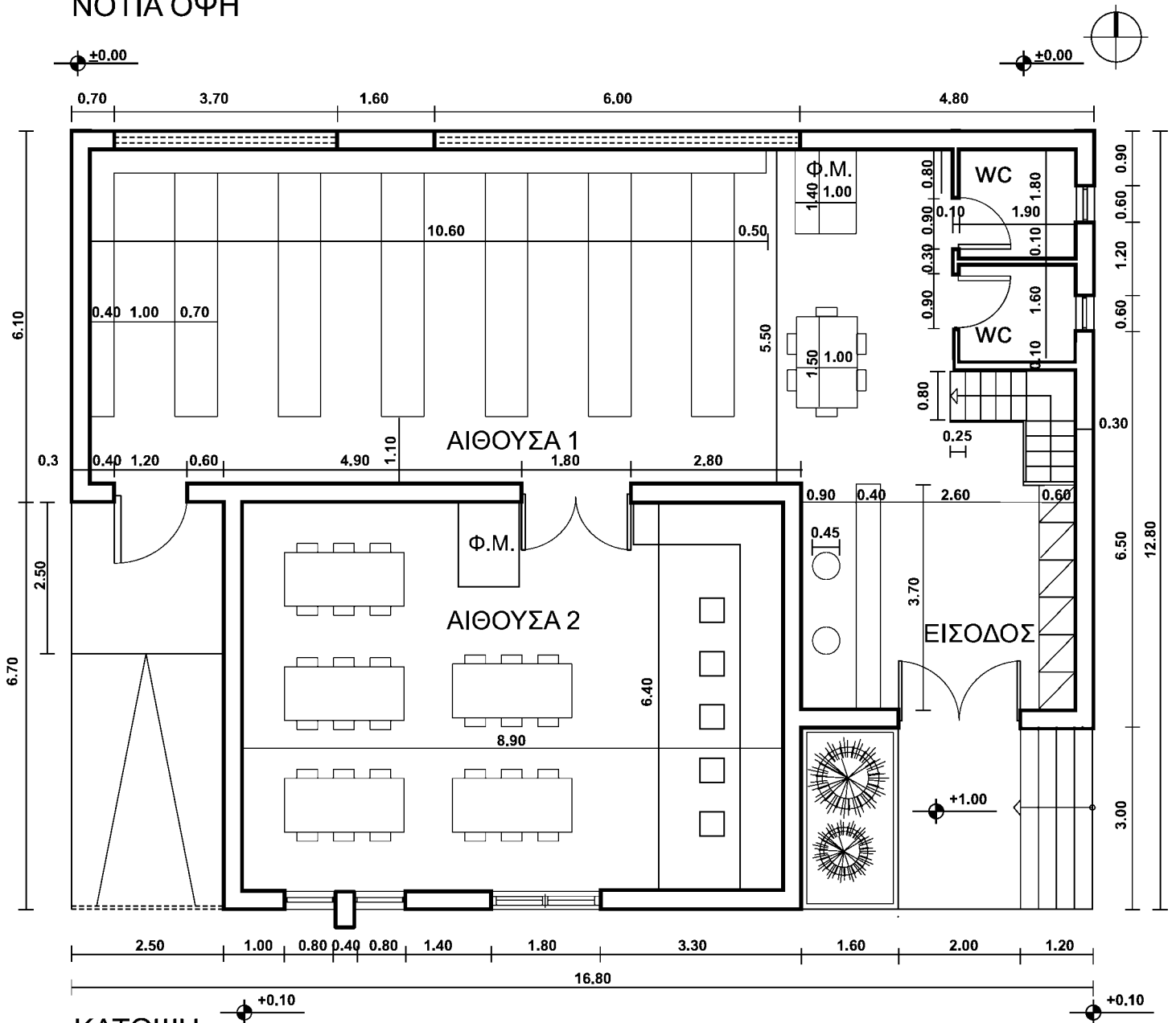
ΚΑΤΟΨΗ
