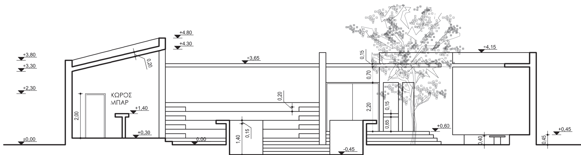
ΤΟΜΗ T-T'
